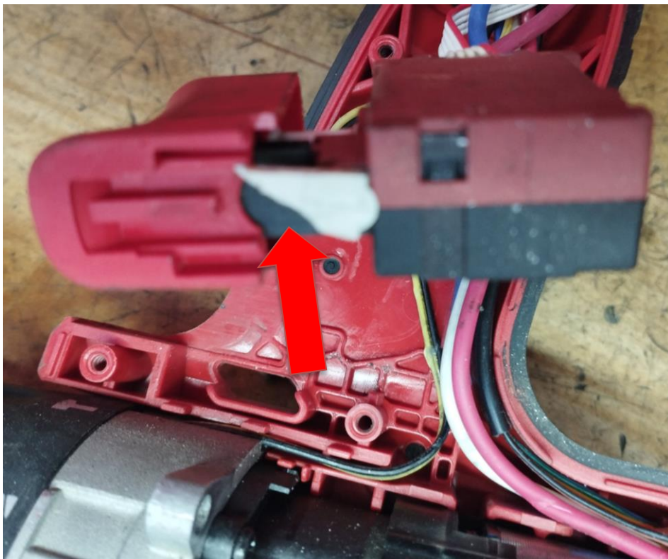
Obr.2 Poškodenie tiahla prepínača smeru otáčok
