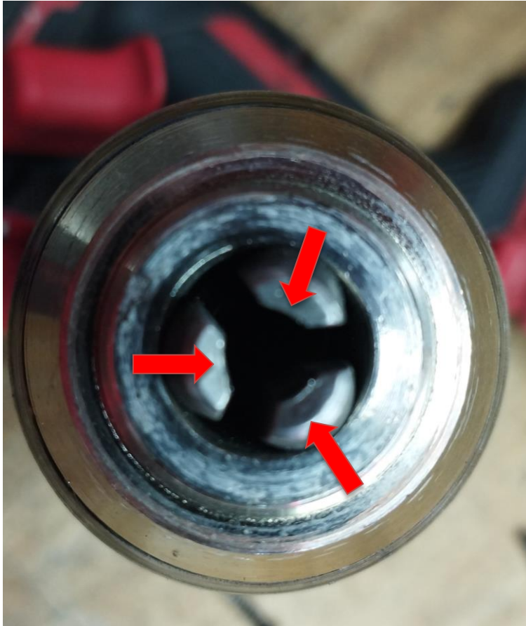
Obr.3 Opatrebenie čeľustí skľučovadla
