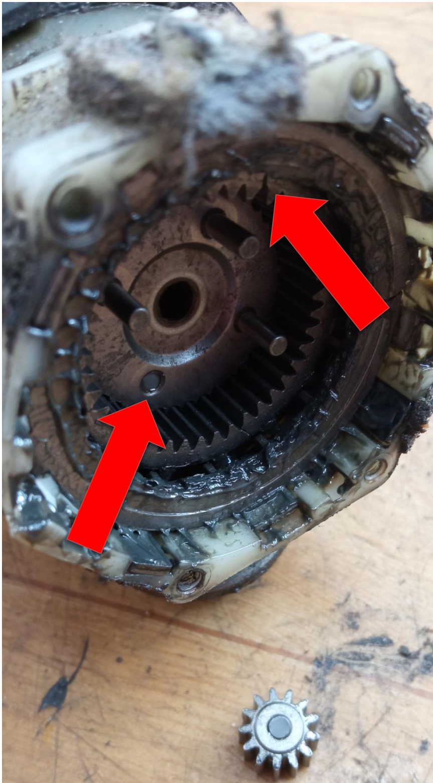
Obr.3 Ulomenie vodiaceho kolíka ozubeného prevodu, poškodenie ozubeného súkolia
