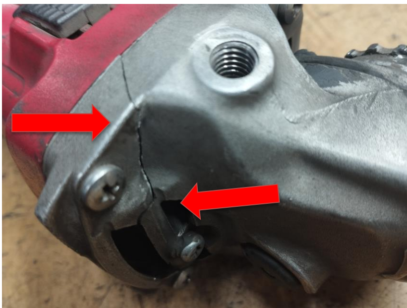
Obr.2 Prasknutie puzdra prevodovky
